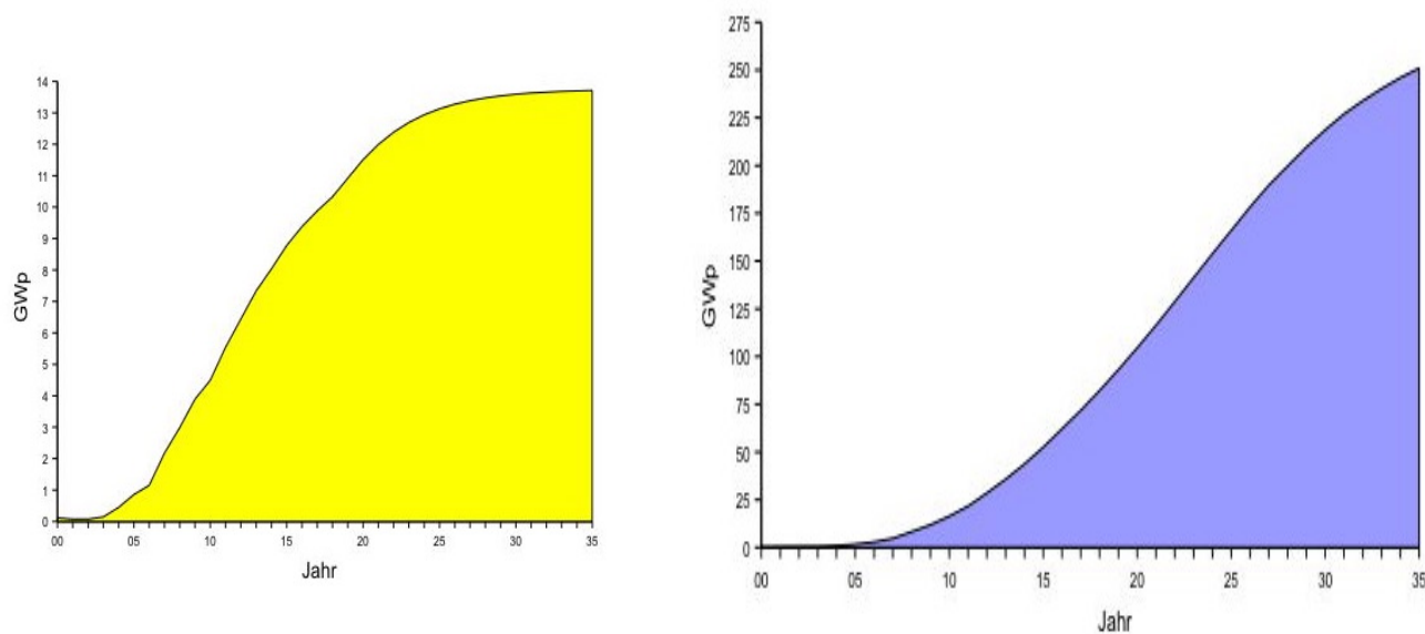
Abbildung 1: Links: Jährlicher Photovoltaik-Zubau; rechts: insgesamt installierte Photovoltaik-Leistung in der Bundesrepublik, jeweils bis 2019 gemäß dem ambitioniertesten der „Photon“-Szenarien, danach auf einer logistischen Kurve, die sich einer jährlichen Installation von 13,75 GWp nähert, entsprechend insgesamt 275 GWp installierter Leistung im Endausbauzustand
