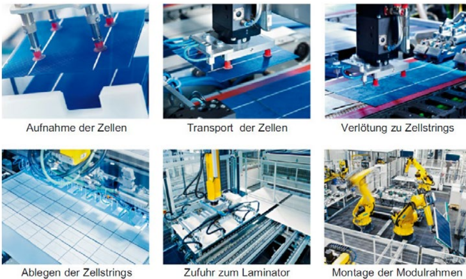
Abb 05 — 9 Fertigungsschritte zur Herstellung eines Solarmoduls (Fotos: Solar-Fabrik AG) •
