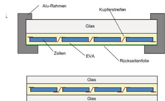
Abb 04 — Aufbau eines Glas-Folien-Moduls (oben) sowie eines Glas-Glas-Moduls (unten) •
