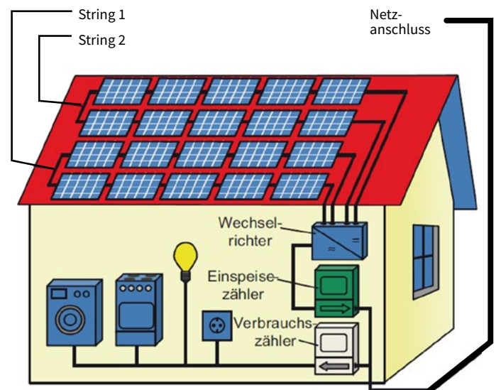
Abb 06 — Aufbau einer typischen netzgekoppelten PV-Anlage •
