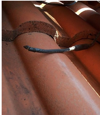
Abb 3 — Strangunterbrechungen können durch Tierbisse vorkommen oder durch nicht fachgerecht verschlossene Steckerverbindungen. •
