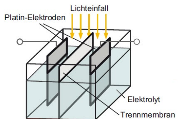
Abb 01 — Versuchsaufbau von Becquerel •
