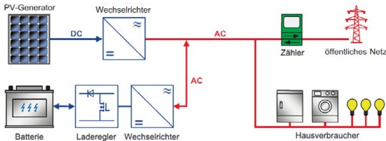
Abb 08 — Prinzipieller Aufbau einer netzgekoppelten Photovoltaikanlage mit Batteriespeicher: a) DC-Kopplung, b) AC-Kopplung •
