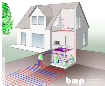
Abb 5 — Flächenkollektor - Wärmepumpe: Es gibt verschiedene Varianten, z.B. Graben-, Ringgraben-, oder Boden-Kollektoren. In ca. 2 m Tiefe werden schlangenförmig Rohre verlegt. Die Wärme wird der Erde entzogen. •
