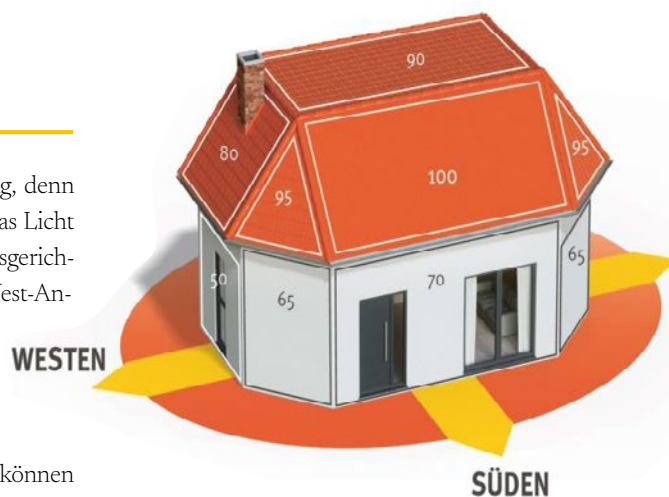
Abb 01a — Die Grafik zeigt, wie viel Prozent Leistung Photovoltaikanlagen auf den verschiedenen Dachflächen und Hauswänden in Relation zu einer Süddachanlage erreichen können. Quelle: Verbraucherzentrale •
