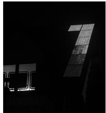
Abb 9 — Das Bild zeigt eine Elektrolumineszenzaufnahme einer PV-Anlage, die vom PID Effekt betroffen ist.
