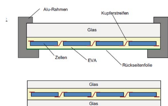
Abb 04 — Aufbau eines Glas-Folien-Moduls (oben) sowie eines Glas-Glas-Moduls (unten) •
