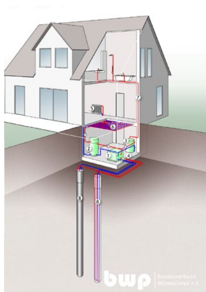
Abb 4 — Geothermie-Wärmepumpe: Über eine Tiefenbohrung von ca. 100m und Erdwärmesonden kann der Erde Wärme entnommen werden •
