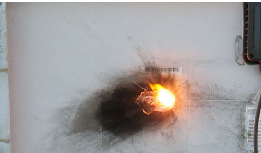
Abb 1 — Problem: versagende Löt- oder Klemmverbindungen innerhalb des Solarmoduls. Das Bild zeigt, wie sich an einem offenen Zellverbinder Mikrolichtbögen bilden, die zur Entzündung der Rückseitenfolie führen.
