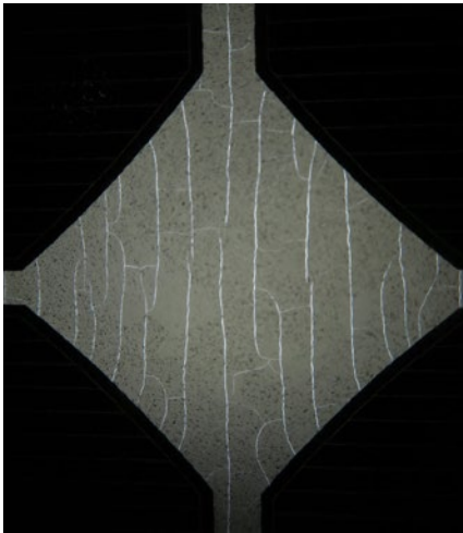
Abb 2 — In einem frühen Stadium lassen sich Isolationsfehler durch die Beleuchtung des Moduls mit einer hellen LED-Lampe erkennen. •
