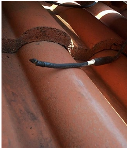
Abb 3 — Strangunterbrechungen können durch Tierbisse vorkommen oder durch nicht fachgerecht verschlossene Steckverbindungen. •
