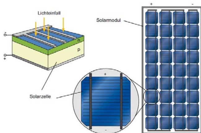
Abb 03 — Solarzelle und Solarmodule als Grundbausteine der Photovoltaik •
