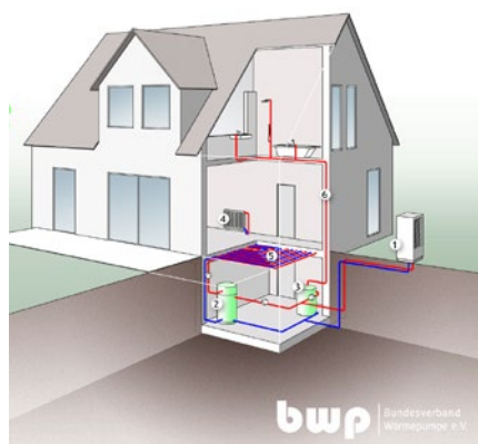
Abb 3 — Luft-Wasser-Wärmepumpe: Der Außenluft wird Wärme entnommen und so der Wasserkreislauf des Heizsystems aufgeheizt. Grafiken: Bundesverband Wärmepumpe (BWP) e.V. •
