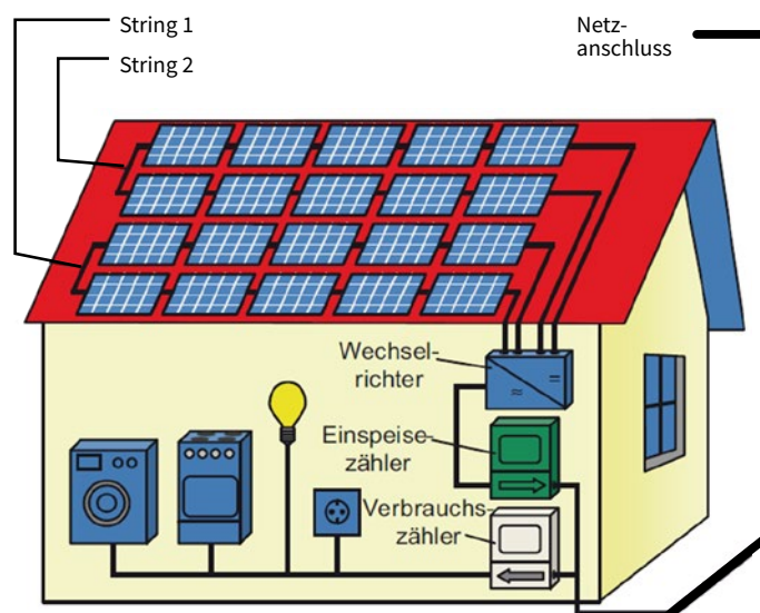
Abb 06 — Aufbau einer typischen netzgekoppelten PV-Anlage •
