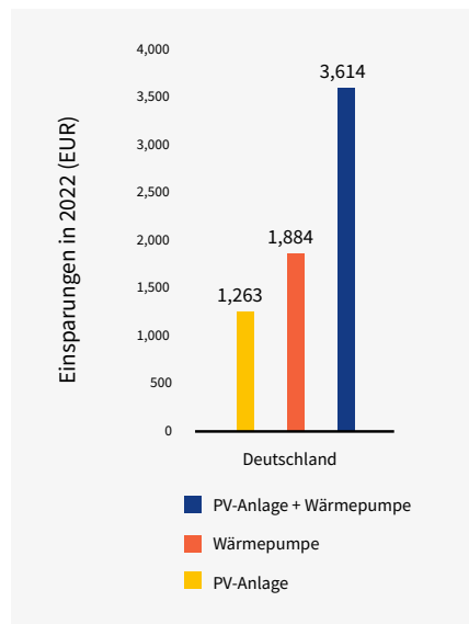
Abb 8 — Laut Solarpower Europe sind die jährlichen Einsparungen in der Wärme- und Stromversorgung durch den kombinierten Einsatz von PV-Anlage und Wärmepumpe am größten •
