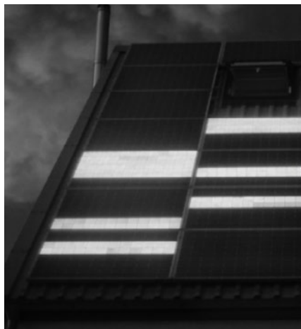
Abb 7 — Das Bild zeigt eine Elektrolumineszenzaufnahme einer Photovoltaikanlage nach einem Überspannungsereignis. Ein Großteil der Bypassdioden sind kurzgeschlossen.
