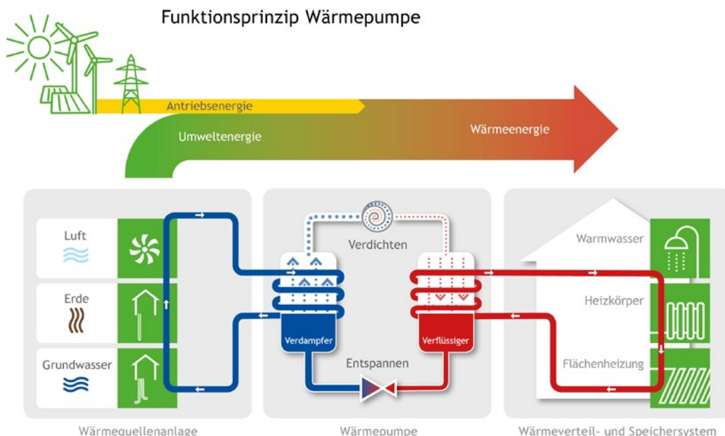
Abb 2 — Funktionsprinzip einer Wärmepumpe: Als Wärmequelle dient die Außenluft oder Sole, die im Erdreich erwärmt wird (links). In der Wärmepumpe (Mitte) wird die Wärme im Verdampfer an das Kältemittel übertragen. Durch Druckerhöhung wird das Kältemittel verflüssigt, welches die Wärme an den Heizungskreislauf des Hauses (rechts) abgibt. Grafik: Bundesverband Wärmepumpe (BWP) e.V. •
