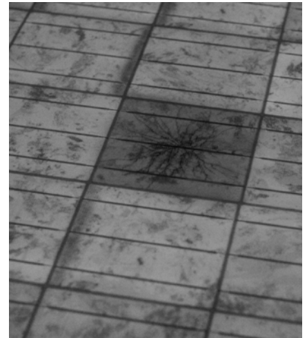
Abb 4 — Das Bild zeigt die Elektrolumineszenzaufnahme eines Solarmoduls mit einem für Hagelschäden typischen Spinnenriss. •
