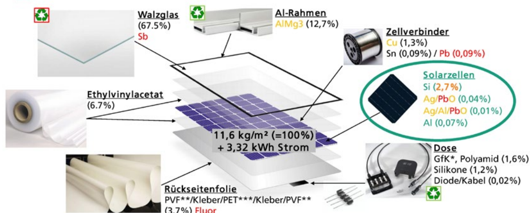
Abb 2 — In Klammern angegeben ist der Massenanteil der Substanz bezogen auf die Gesamtmodulmasse von 11,6 kg/m 2 . *GfK Glasfaser verstärkter Kunststoff, **PVF Polyvinylfluorid, ***PET Polyethylenterephthalat © Fraunhofer ISE.
