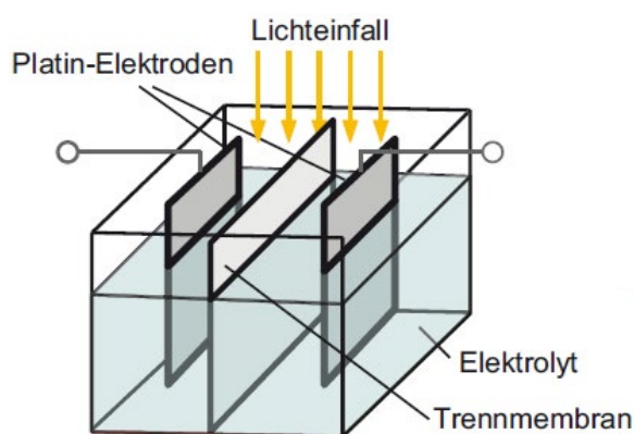
Abb 01 — Versuchsaufbau von Becquerel •
